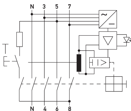
Anschlussschema DFS 4 B SK MI HD, 4-polig
