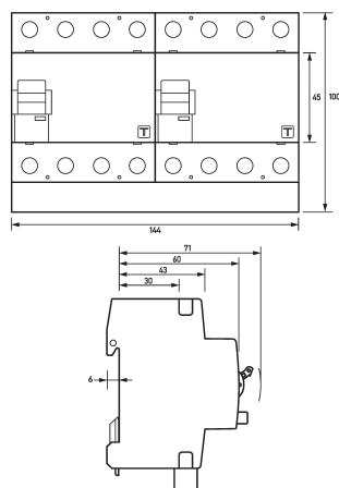
Dibujo acotado DFS 4 A Twin, 4 polos (Vista de grupos)
