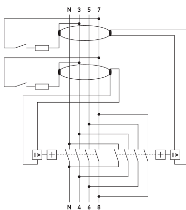
Esquema de conexiones DFS 4 A Twin, 4 polos
