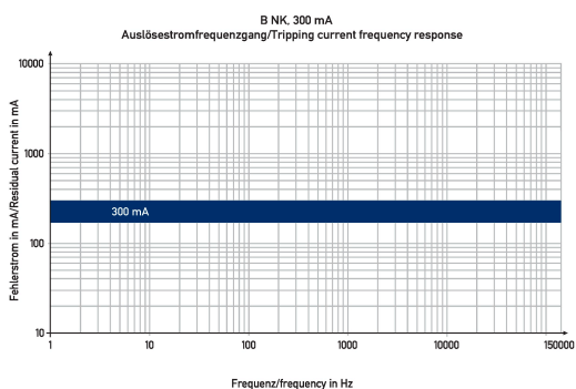
Diagramme Fehlerstromschutzschalter DFS 4 040-2/0,30-B NK
