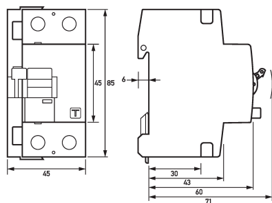
Maßzeichnung Fehlerstromschutzschalter DFS 2 040-2/0,30-A FT
