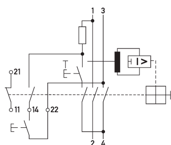
Schaltungsbeispiel Fehlerstromschutzschalter DFS 2 040-2/0,30-A FT
