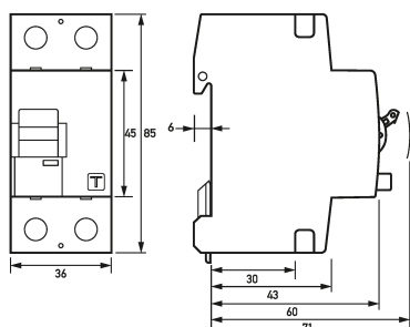
Dibujo acotado Interruptores diferenciales DFS 2 040-2/0,30-A
