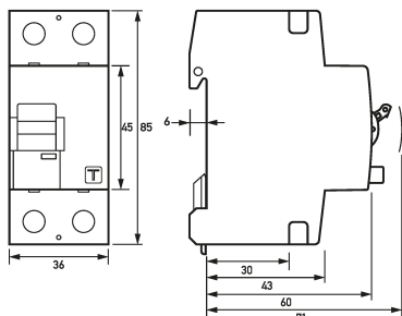
Maßzeichnung Fehlerstromschutzschalter DFS 2 040-2/0,3-A HD
