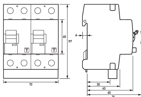
Dibujo acotado Interruptores diferenciales DFS 2 040-2/0,30-A Twin
