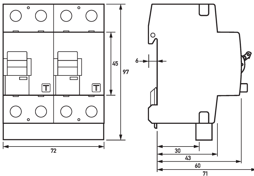
Dibujo acotado DFS 2 A KV Twin, 2 polos (Vista de grupos)
