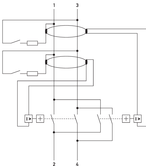
Esquema de conexiones DFS 2 A KV Twin, 2 polos
