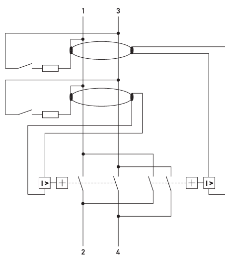
Schaltungsbeispiel Fehlerstromschutzschalter DFS 2 040-2/0,30-A KV Twin
