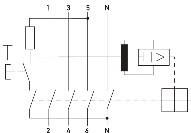
Esquema de conexiones DFS 4 A, 4 polos N derecha
