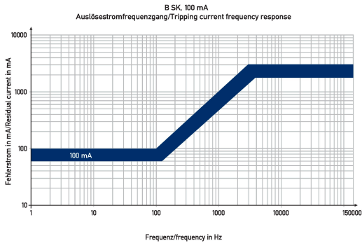
Curva característica B SK 100 mA
