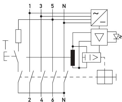
Schaltungsbeispiel Fehlerstromschutzschalter DFS 4 040-4/0,10-PV R HD
