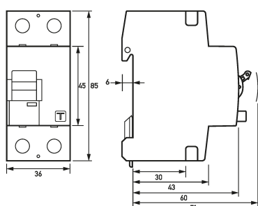
Maßzeichnung Fehlerstromschutzschalter DFS 2 040-2/0,10-PV
