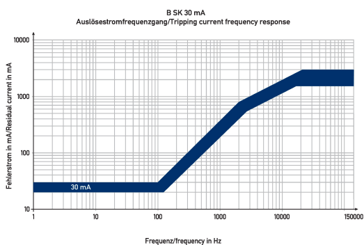
Diagramme Fehlerstromschutzschalter DFS 4 040-4/0,03-B SK V500
