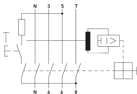
Schaltungsbeispiel Fehlerstromschutzschalter DFS 4 040-4/0,03-A KV V500 HD
