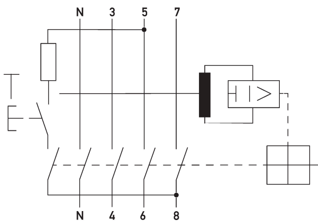
Anschlussschema DFS 4 A Hz400, 4-polig
