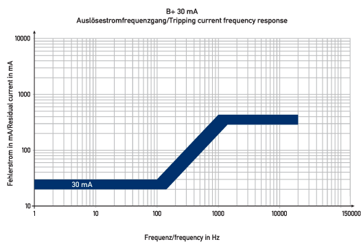
Diagramme Fehlerstromschutzschalter DFS 4 040-4/0,03-B+
