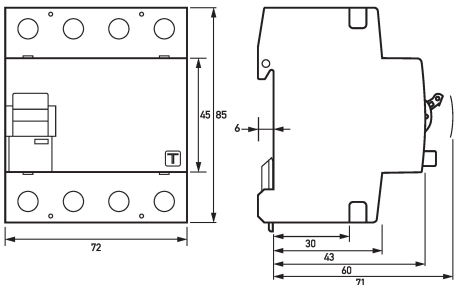
Maßzeichnung Fehlerstromschutzschalter DFS 4 040-4/0,03-B SK MI HD
