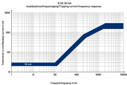
Diagramme Fehlerstromschutzschalter DFS 4 040-4/0,03-B SK MI HD
