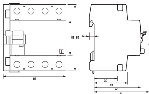
Maßzeichnung Fehlerstromschutzschalter DFS 4 040-4/0,03-A ASAO 12
