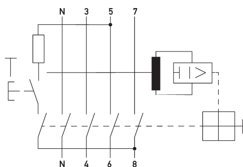
Schaltungsbeispiel Fehlerstromschutzschalter DFS 4 040-4/0,03-F
