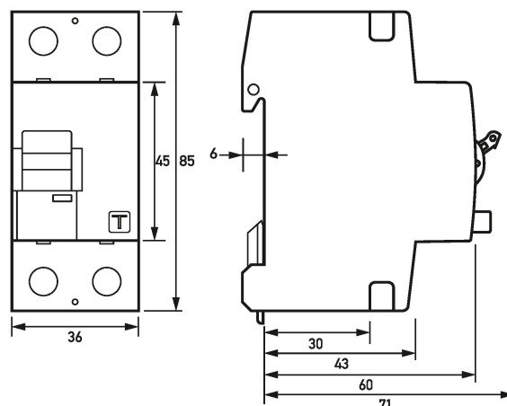
Dibujo acotado DFS 2 A KV HD, 2 polos (Vista de grupos)
