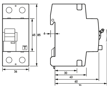
Maßzeichnung Fehlerstromschutzschalter DFS 2 040-2/0,03-A V24
