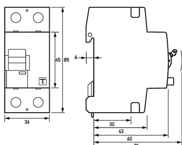
Dibujo acotado Interruptores diferenciales DFS 2 040-2/0,03-A HD
