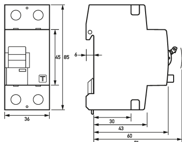
Maßzeichnung Fehlerstromschutzschalter DFS 2 040-2/0,01-A V110
