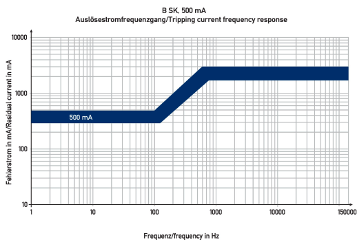
Curva característica B SK 500 mA
