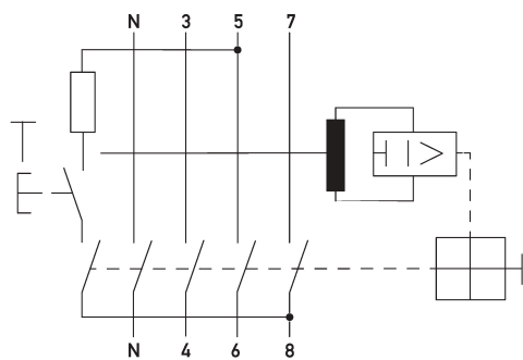
Ejemplo de cableado Interruptores diferenciales DFS 4 025-4/0,50-A
