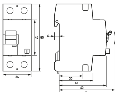
Dibujo acotado Interruptores diferenciales DFS 2 025-2/0,50-A
