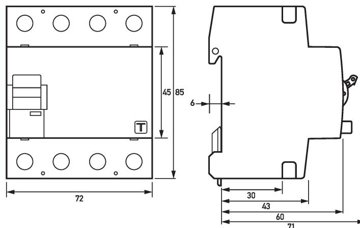
Dibujo acotado DFS 4 B SK V500, 4 polos (Vista de grupos)
