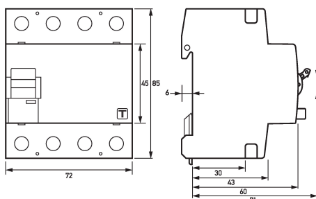
Maßzeichnung Fehlerstromschutzschalter DFS 4 025-4/0,30-A V500
