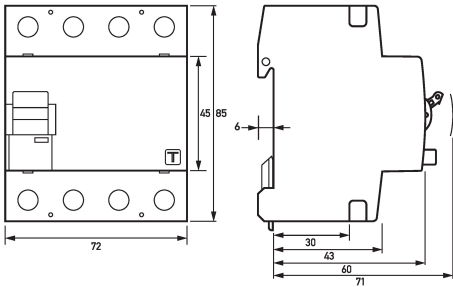
Dibujo acotado Interruptores diferenciales DFS 4 025-4/0,30-B+ MI HD
