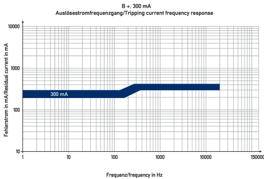
Diagramas Interruptores diferenciales DFS 4 025-4/0,30-B+ MI HD
