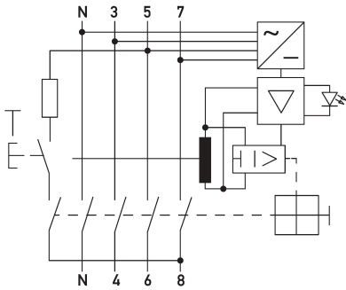
Ejemplo de cableado Interruptores diferenciales DFS 4 025-4/0,30-B+ MI HD
