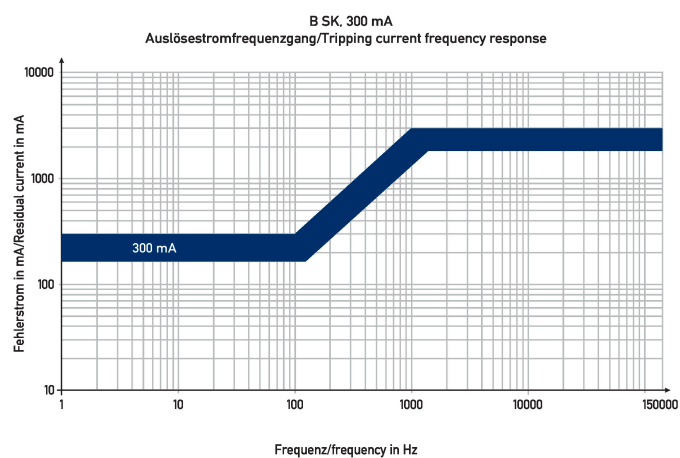
Curva característica B SK 300 mA
