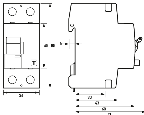
Dibujo acotado DFS 2 A, 2 polos (Vista de grupos)
