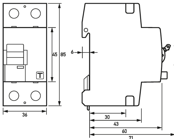
Maßzeichnung DFS 2 A HD, 2-polig (Gruppenansicht)
