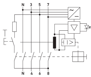
Anschlussschema
