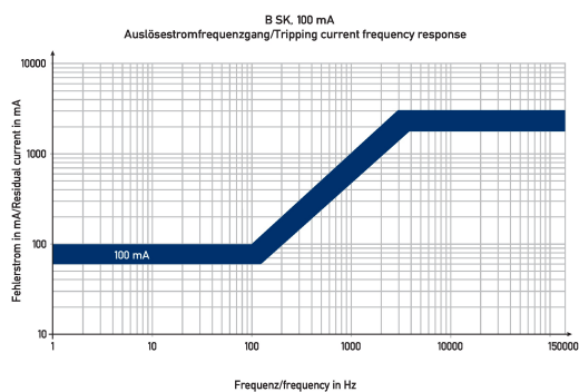
Diagramme Fehlerstromschutzschalter DFS 4 025-4/0,10-B SK V500
