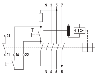
Schaltungsbeispiel Fehlerstromschutzschalter DFS 4 025-4/0,10-A FT
