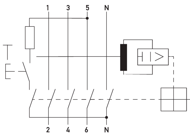
Esquema de conexiones DFS 4 A HD, 4 polos N derecha
