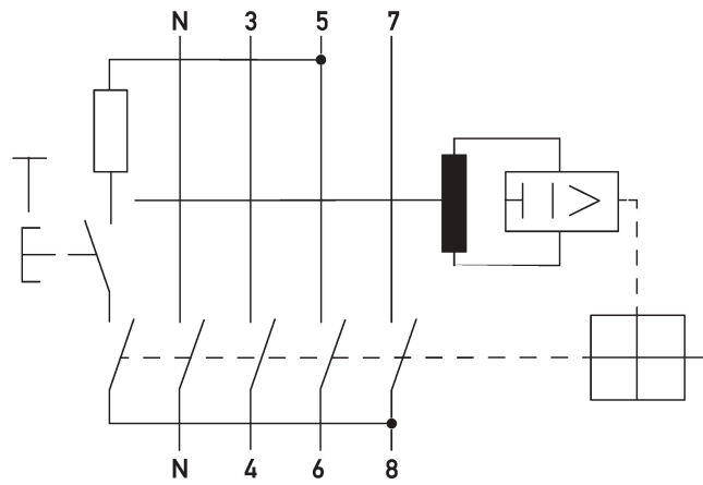
Anschlussschema DFS 4 AC, 4-polig
