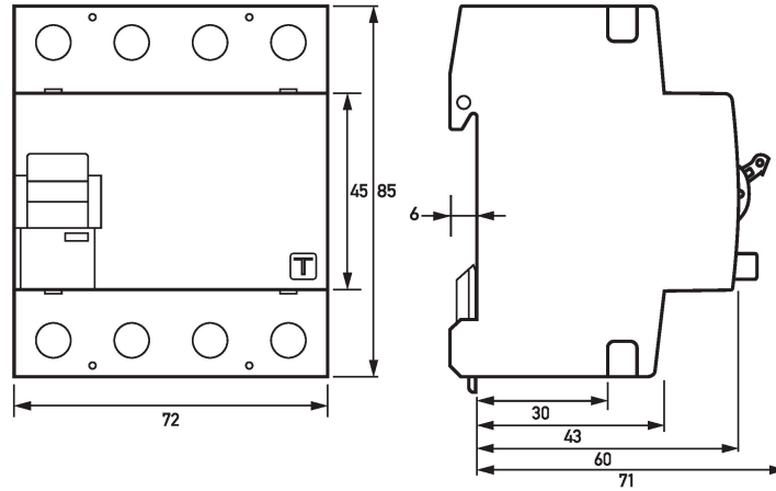
Maßzeichnung DFS 4 AC, 4-polig (Gruppenansicht)
