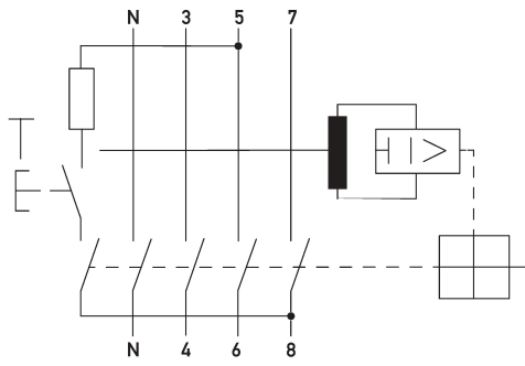
Schaltungsbeispiel Fehlerstromschutzschalter DFS 4 025-4/0,03-A HD
