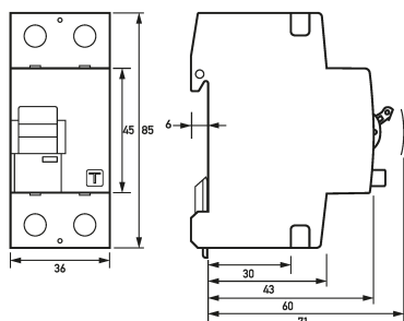
Maßzeichnung Fehlerstromschutzschalter DFS 2 025-2/0,03-A
