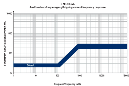
Curva característica B NK 30 mA
