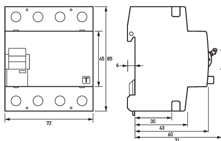
Maßzeichnung Fehlerstromschutzschalter DFS 4 025-2/0,03-A EV
