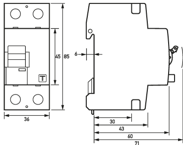
Dibujo acotado Interruptores diferenciales DFS 2 025-2/0,01-A
