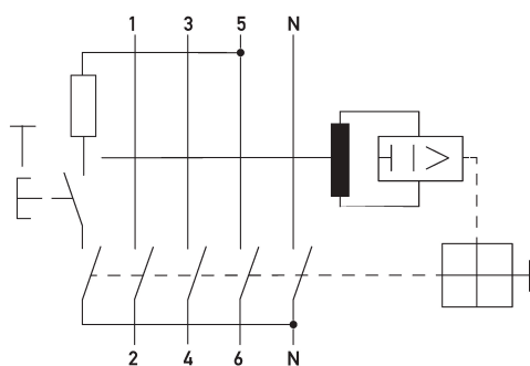
Schaltungsbeispiel Fehlerstromschutzschalter DFS 4 016-4/0,30-A KV R HD
