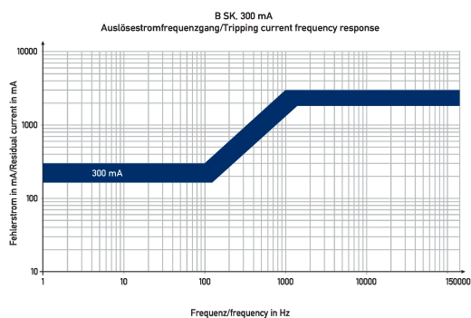
Diagramme Fehlerstromschutzschalter DFS 4 016-4/0,30-B SK NA
