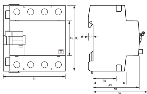
Mazeichnung Fehlerstromschutzschalter DFS 4 016-4/0,30-B SK NA
