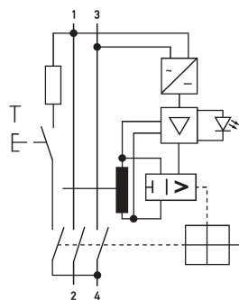
Anschlussschema DFS 2 B SK HD, 2-polig
