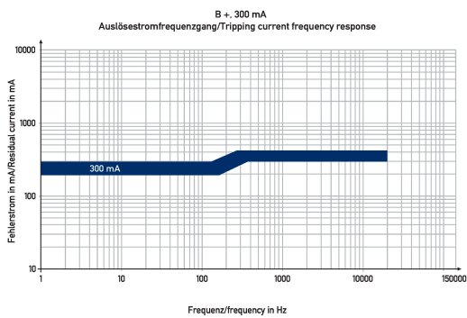
Curva característica B+ 300 mA
