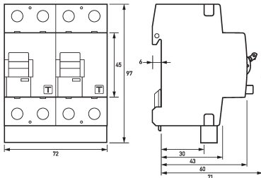
Maßzeichnung Gruppenansicht
