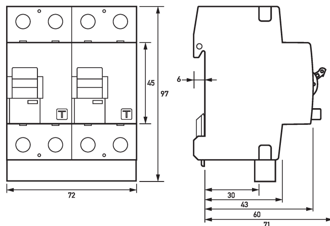
Dibujo acotado DFS 2 A Twin, 2 polos (Vista de grupos)
