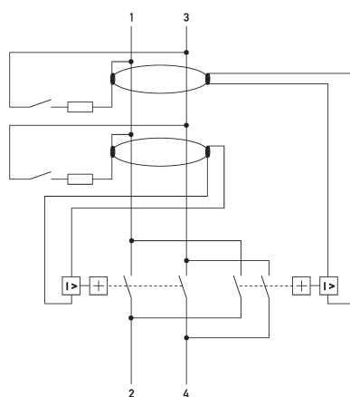
Esquema de conexiones DFS 2 A Twin, 2 polos
