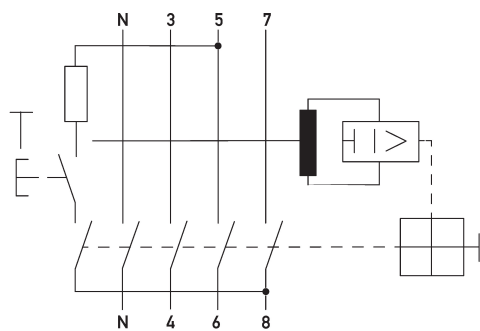
Ejemplo de cableado Interruptores diferenciales DFS 4 016-4/0,10-A
